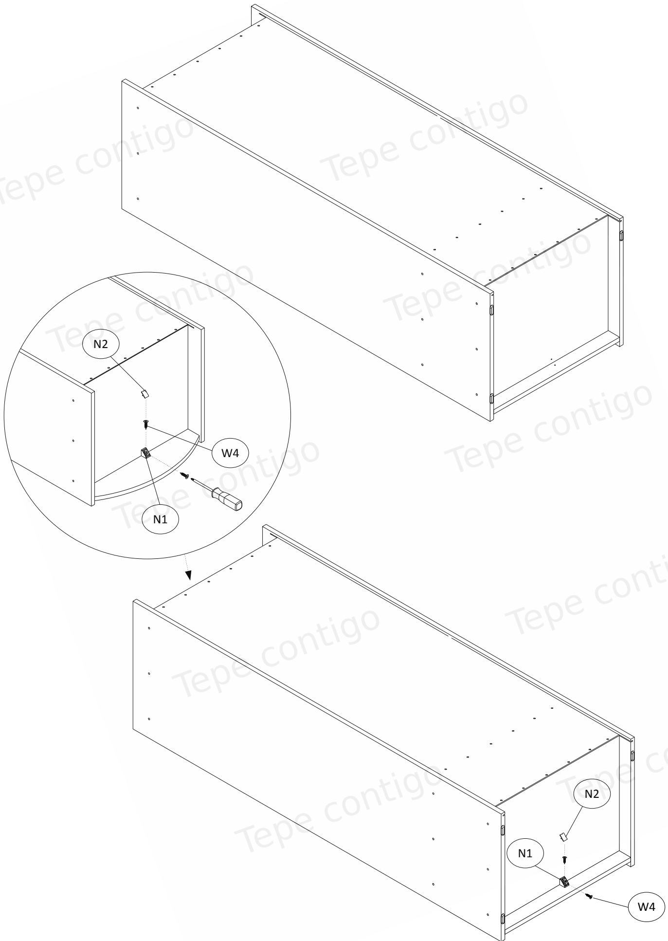
Skřín SZ05-A L / Wardrobe SZ05-A L
